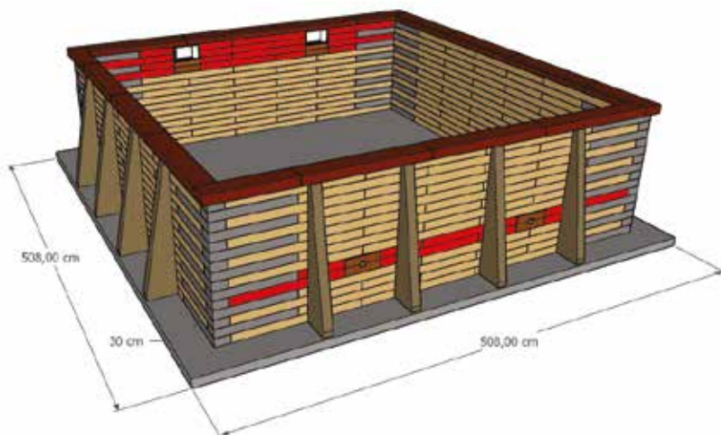
POSE HORS-SOL/SEMI-ENTERRÉE (1/3 ENTERRÉE) 16X RENFORTS OBLIGATOIRES
