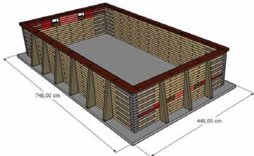
POSE HORS-SOL/SEMI-ENTERRÉE (1/3 ENTERRÉE) 18X RENFORTS OBLIGATOIRES
