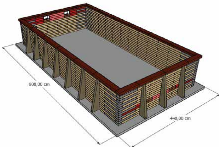
POSE HORS-SOL/SEMI-ENTERRÉE (1/3 ENTERRÉE) 20X RENFORTS OBLIGATOIRES
