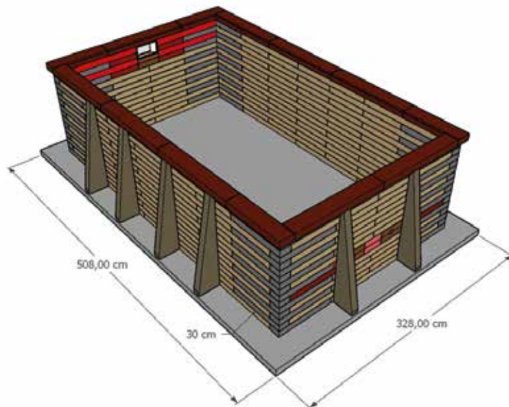
POSE HORS-SOL/SEMI-ENTERRÉE (1/3 ENTERRÉE) 12X RENFORTS OBLIGATOIRES
