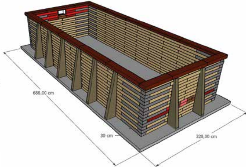
POSE HORS-SOL/SEMI-ENTERRÉE (1/3 ENTERRÉE) 16X RENFORTS OBLIGATOIRES
