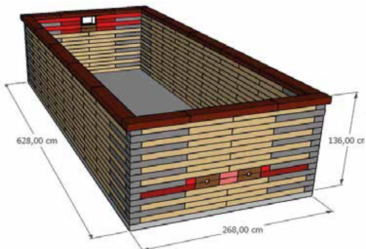
POSE ENTERRÉE/SEMI-ENTERRÉE (2/3 ENTERRÉE)
